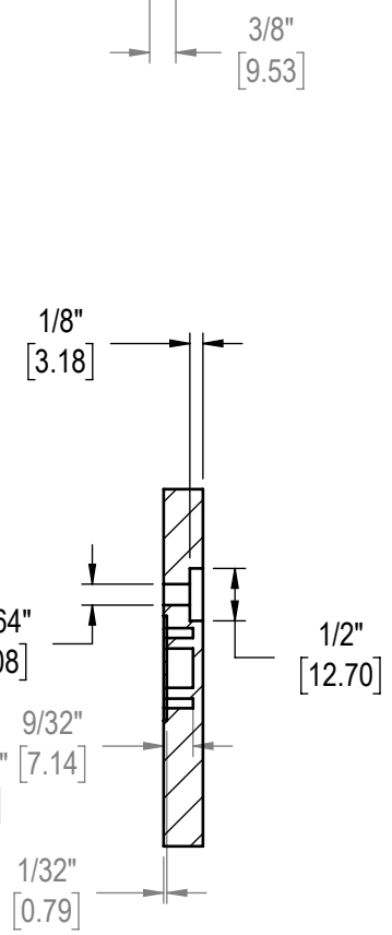
SECTION B-B SCALE 1 : 2
